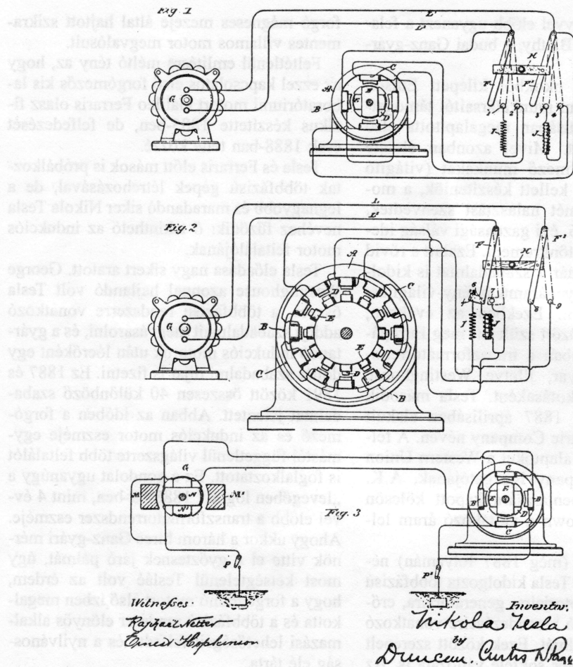
3. ábra A soros kapcsolású induktivitással létesített fáziseltolás szabadalmi rajza
